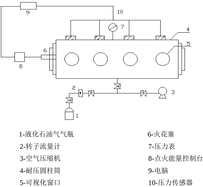
图 1 测试装置示意图
